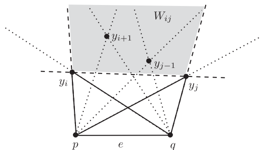
Fig. 10. The region W_{ij} .
